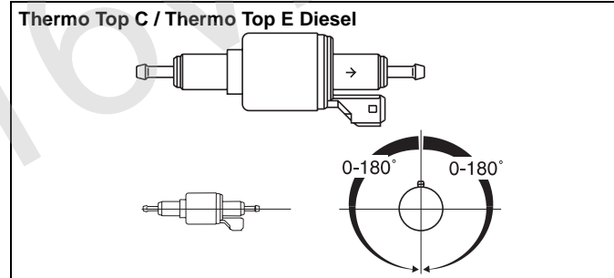
Bild 11: Dosierpumpe DP 30
