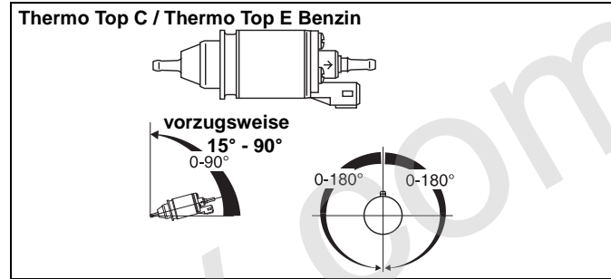
Bild 10: Dosierpumpe DP 2
