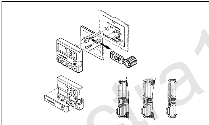
Bild 15: Einbau Vorwähluhr
