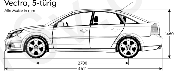
Vectra, 5-türig
