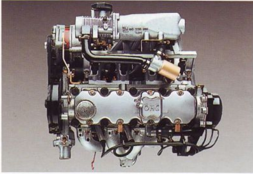
Das 2.0i-Triebwerk mit 85 kW (115 PS) und geregeltm Katalysator.
